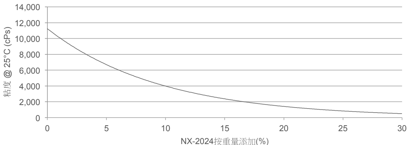
NX-2024与液体环氧树脂混合的稀释曲线图（环氧当量=190）
